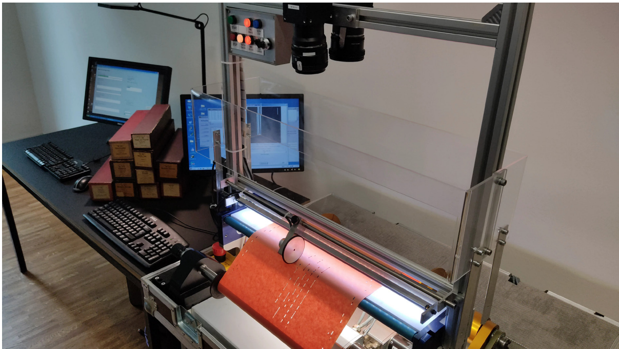
Abb. 2. Der an der BFH-TI entwickelte Musikrollenscanner in den Räumlichkeiten der HKB Forschung. Foto: Sebastian Bausch.
